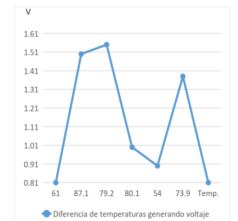
Gráfica 1. Registro de datos Temperatura vs voltaje Héctor Santacruz López 2017
