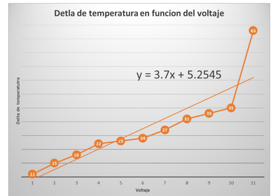
Gráfica 2. Registro de datos Voltaje vs Temperatura Héctor Santacruz López 2017
